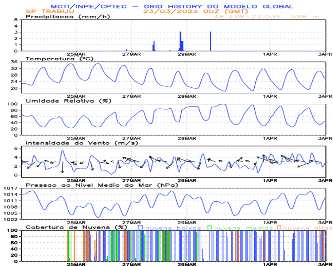
Figura 6. Meteograma do município de Trabiçu com dados de Precipitação, temperatura, UR, vento em 10 m, PNMM e cobertura de nuvens.
